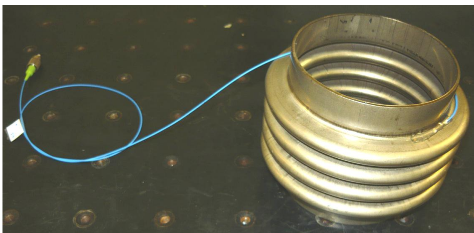
Волоконно-оптический датчик акустический на сильфоне компенсаторе
